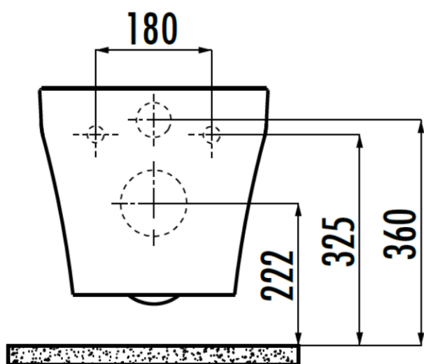
Схема монтажа унитаза без функции биде
