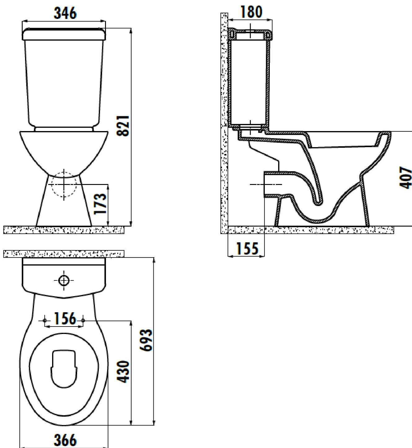
Схема монтажа унитаза
